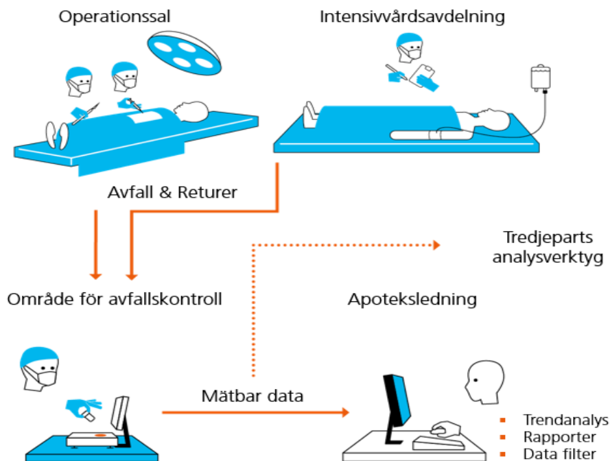
Figur 4 – Arbetsflöde WasteLog™
